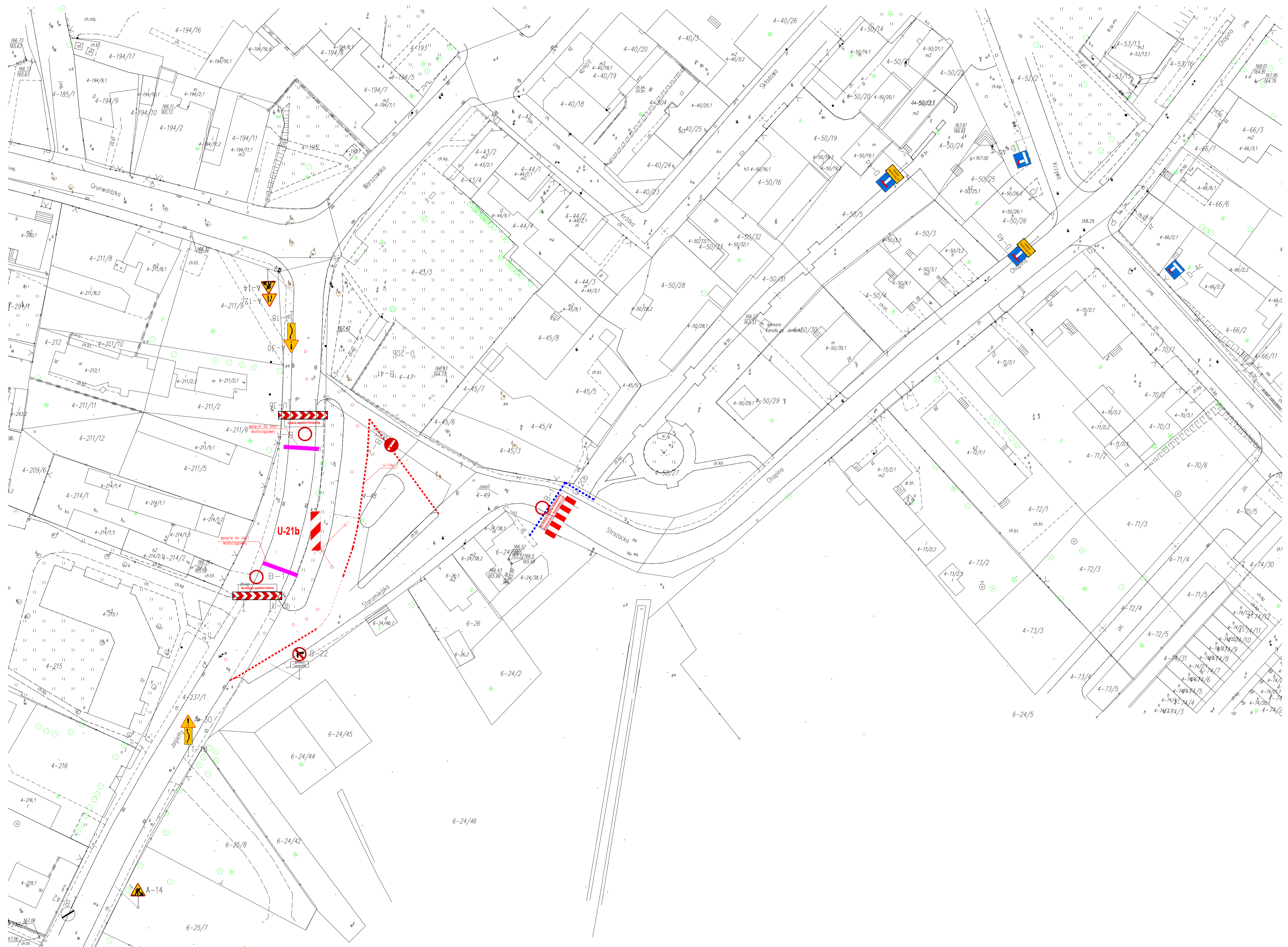
Rys. 2 ETAP I skala 1:500
